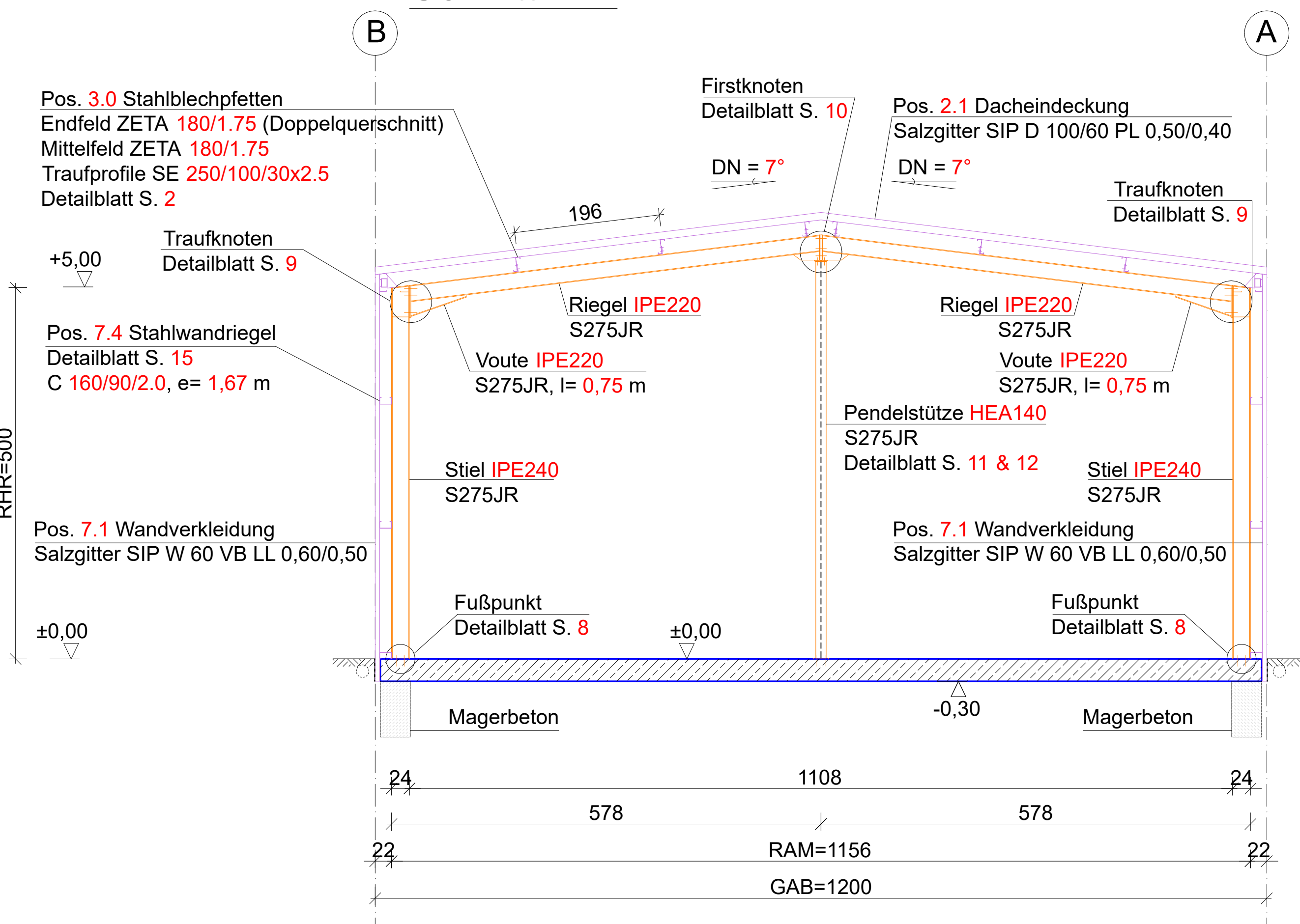
Pos 5.0 Giebelrahmen Achse 1&5 mit PV-Anlage Schnitt A-A
