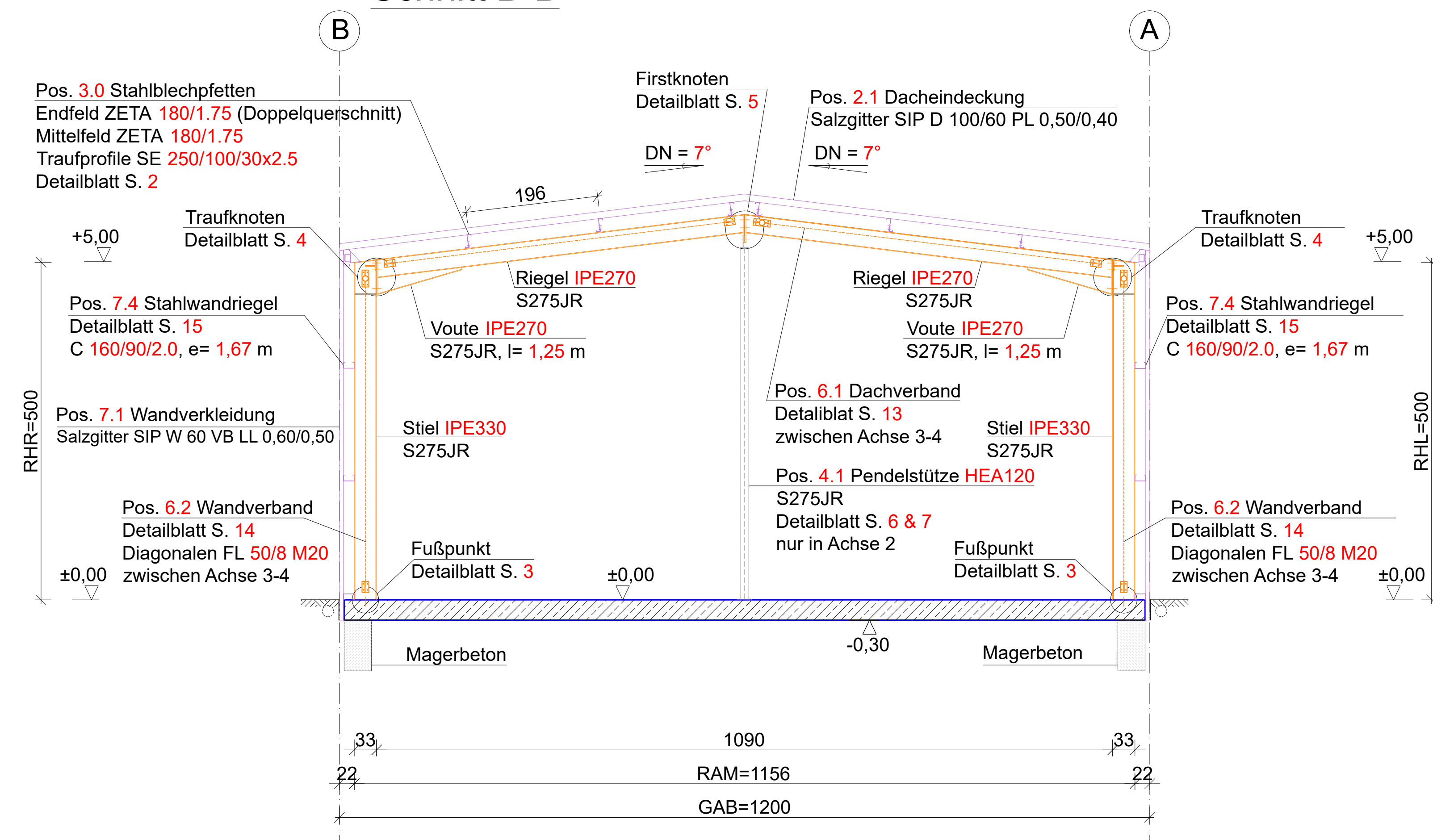
Pos 4.0 Rahmen Achse 2-4 mit PV-Anlage Schnitt B-B
